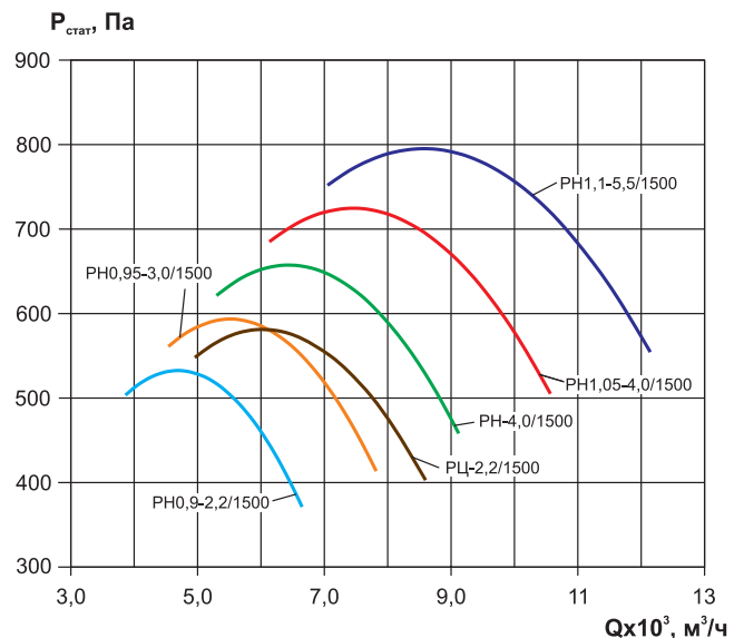
ВКРФ-М-50-РН(РЦ) (1500 об/мин)
