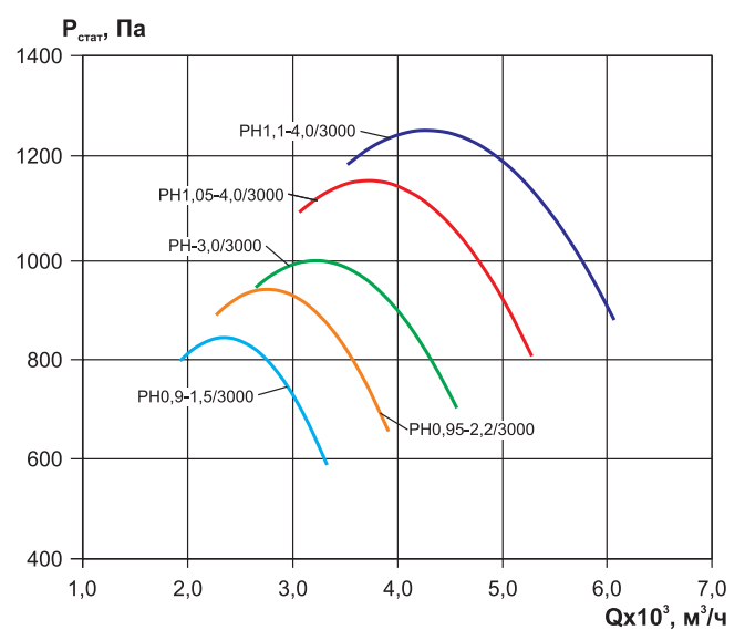
ВКРФ-М-31-РН (3000 об/мин)
