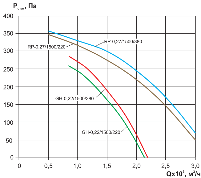
ВКРФ-М-45-GH(RP)
