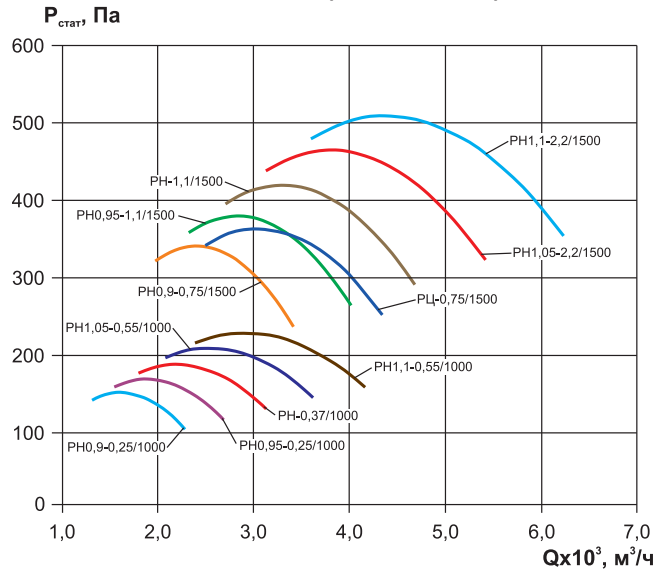
ВКРФ-М-45-РЦ
