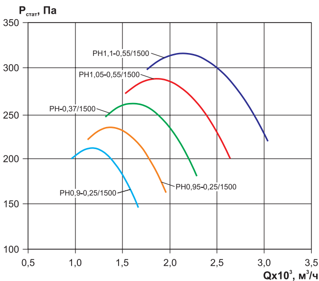
ВКРФ-М-31-РН (1500 об/мин)
