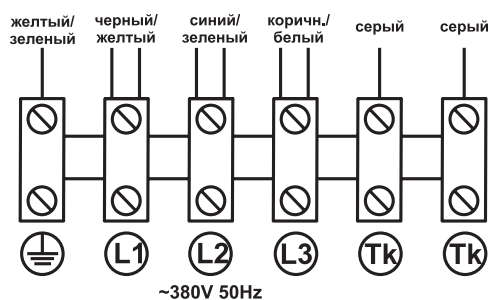
Схема подключения №10
