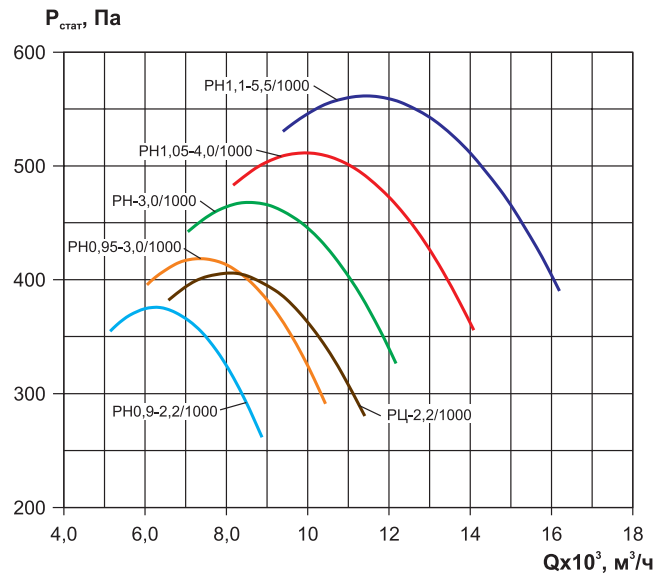
ВКРФ-М-71-РЦ
