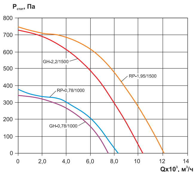
ВКРФ-М-56-GH(RP)
