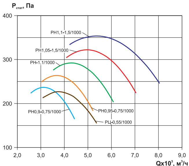
ВКРФ-М-50-РН(РЦ) (1000 об/мин)
