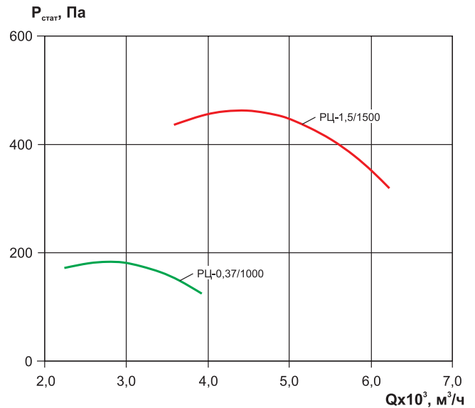
ВКРФ-М-50-РН(РЦ) (1500 об/мин)
