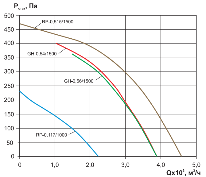
ВКРФ-М-50-GH(RP)
