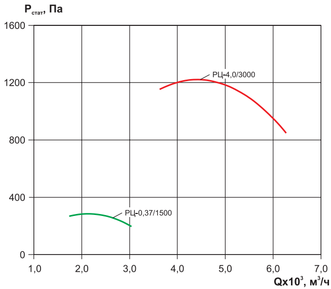
ВКРФ-М-40-РН(РЦ) (3000 об/мин)
