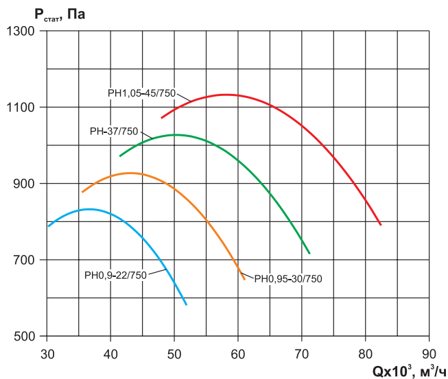
ВКРФ-М-125-РН
