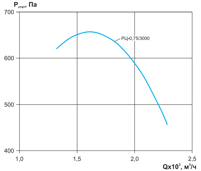
ВКРФ-М-31-РЦ
