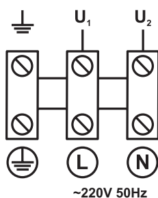
Схема подключения №11
