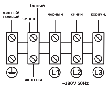
Схема подключения №9
